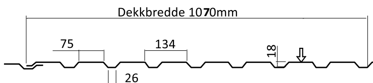
Mål FP18 - stål 0,4mm
