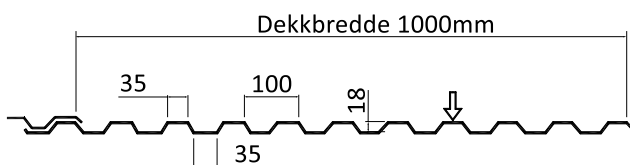
Mål TR 20 - stål 0,5mm
